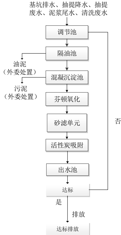
图 7.2-1 污水处理工艺流程
