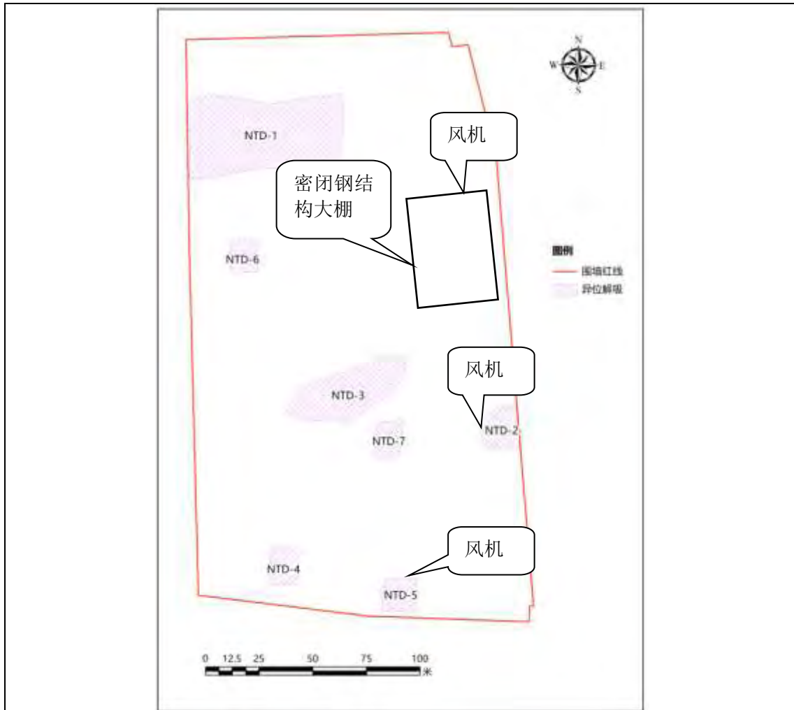
图 7.3-3 第三阶段施工距离最近时噪声分布图
