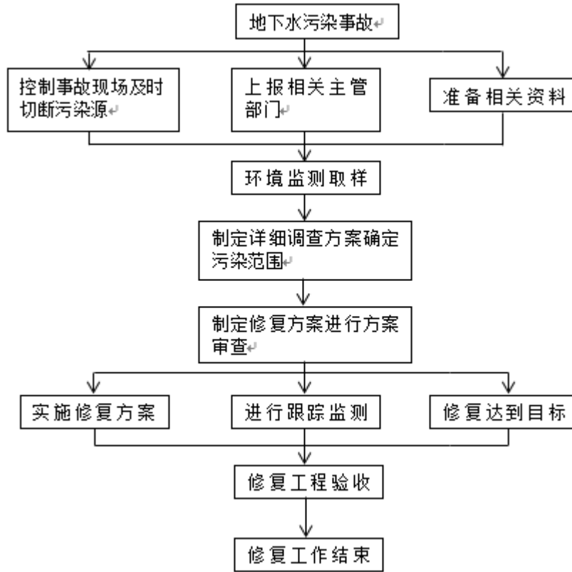
图 7.5-3 应急响应流程图
