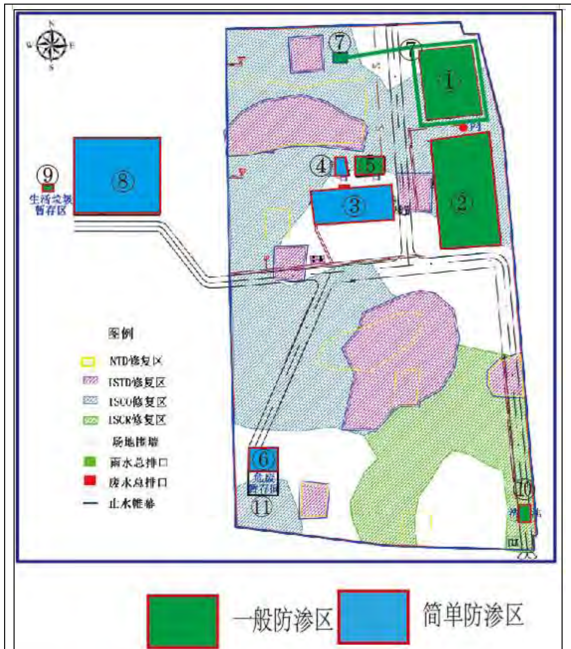
图 7.5-2 本项目防渗分区图
