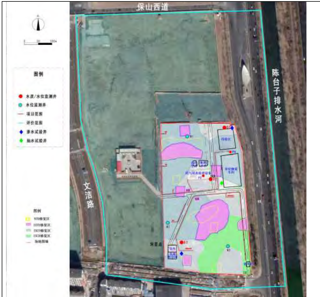
图 7.5-1 地下水评价范围
