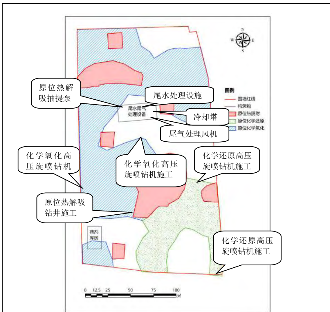
图 7.3-2 第二阶段施工距离最近时主要噪声源分布情况
